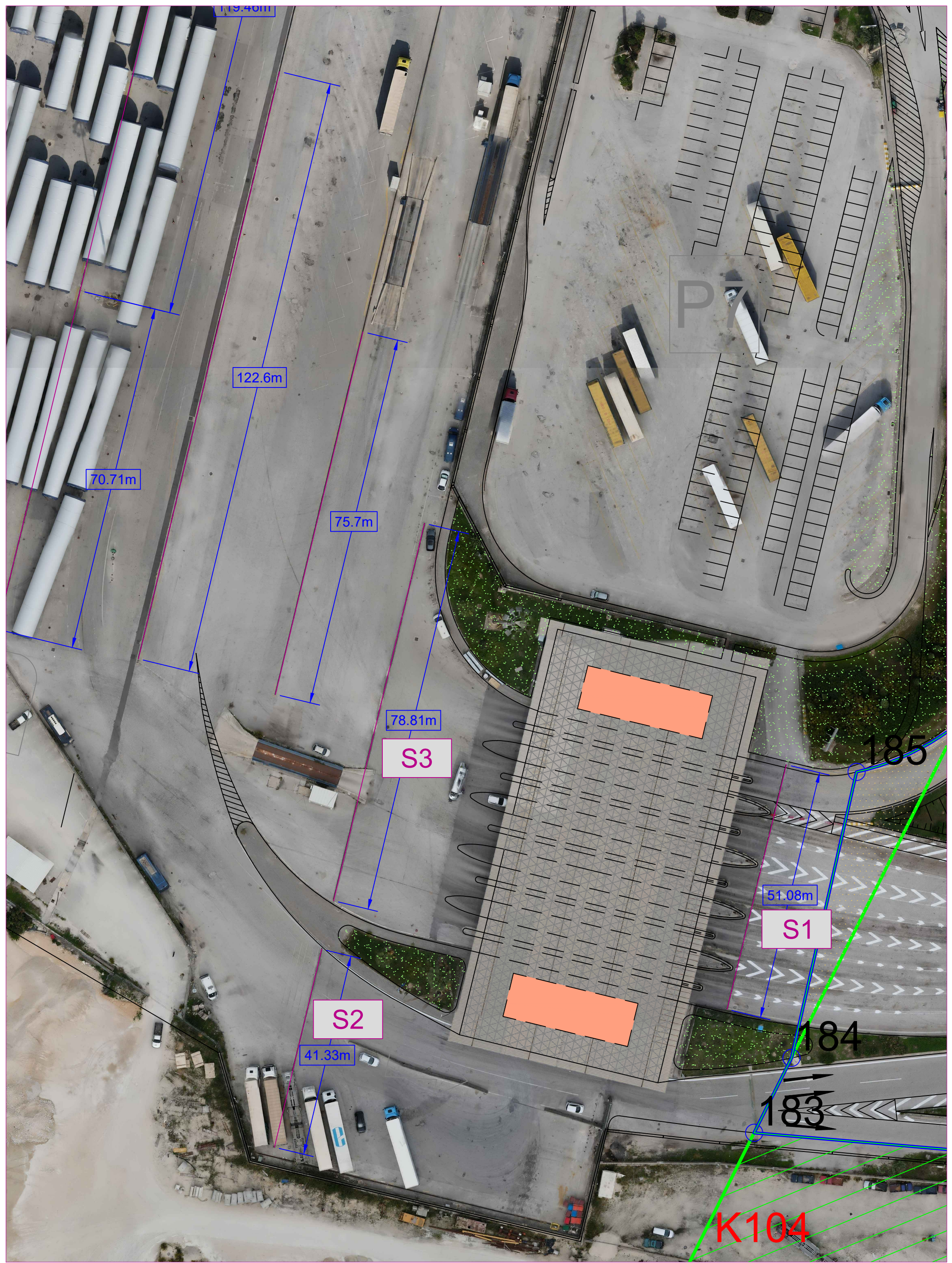
Layout // Water Drainage Channels & Gratings Replacement // Segments S1 - S2- S3 Σχέδιο Διάταξης // Αντικατάσταση Καναλιών Απορροής & Σχαρών // Τμήματα S1 - S2- S3
